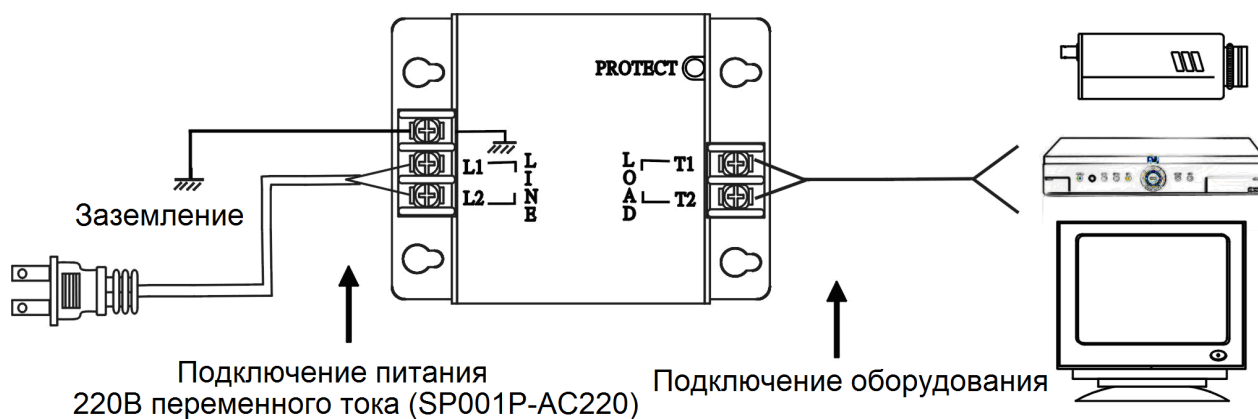
Рис. 2 Схема подключения SP001P-AC220
