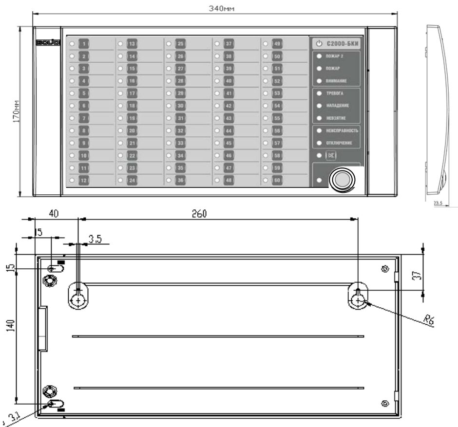
Рисунок 1. Внешний вид, габаритные и установочные размеры блока
