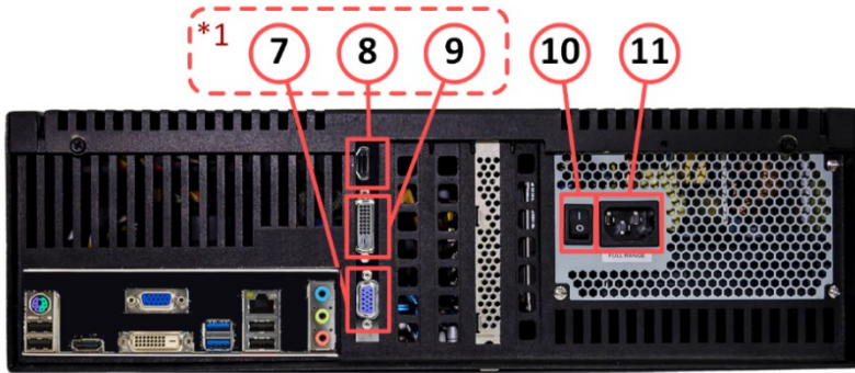
Рисунок 2. Задняя панель
