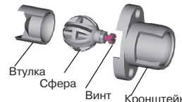
Детали кронштейна
