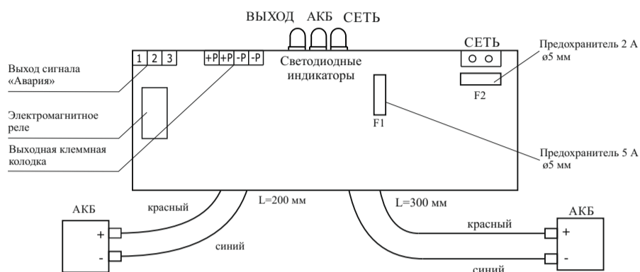
Рисунок 4 – Схема подключения платы БР12
