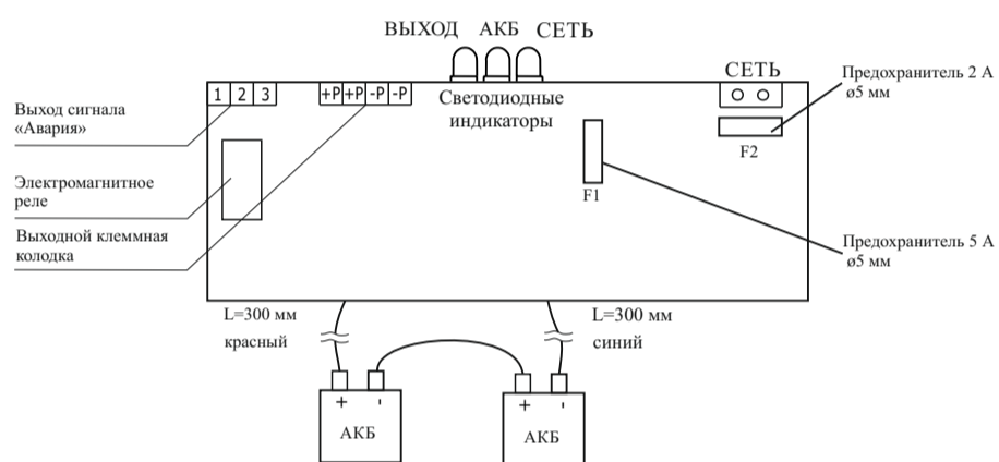
Рисунок 5 – Схема подключения платы БР24
