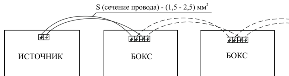
Рисунок 2 – Схема подключения боксов к источнику
