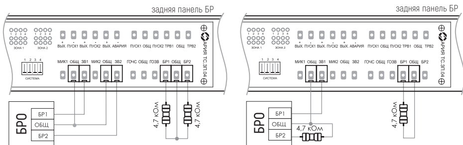
Рис. 22 Подключение блока расширения АРИЯ-ТС-БР-РМ-2-120 к блоку речевого оповещения АРИЯ-ТС-БР0
