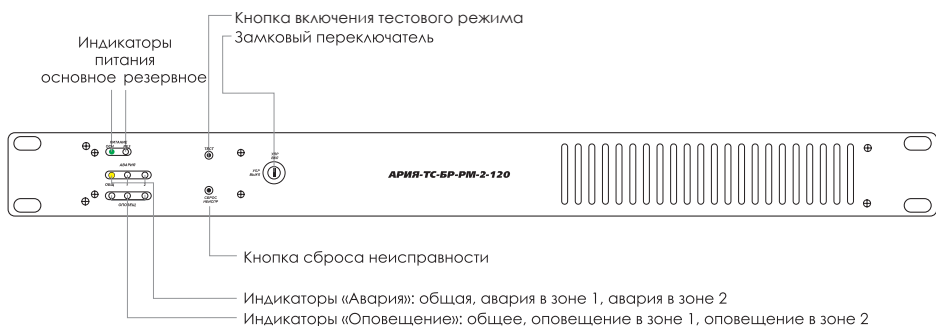
Рис. 28 Передняя панель блока расширения АРИЯ-ТС-БР-PM-2-120
