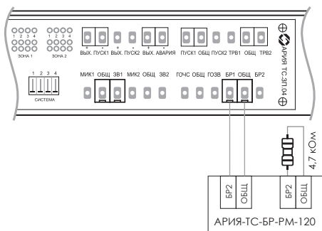
Рис. 4. Подключение дополнительных блоков расширения к АРИЯ-ТС-БР-PM-120
