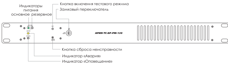
Рис. 12 Передняя панель блока расширения АРИЯ-ТС-БР-РМ-120
