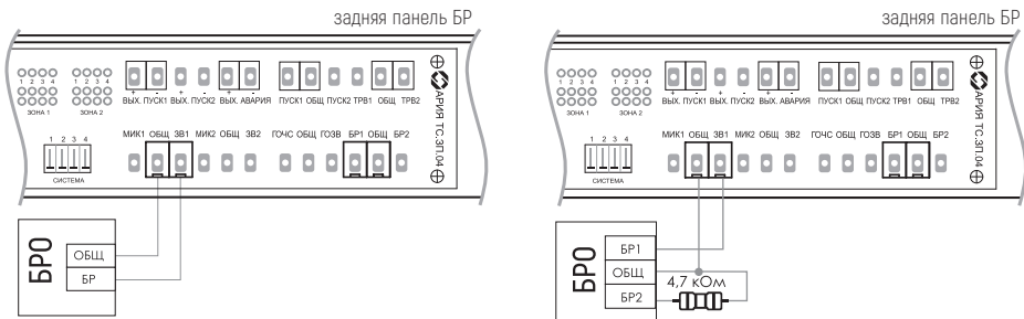
Рис. 3. Подключение блоков расширения АРИЯ-ТС-БР-PM-120 к блоку речевого оповещения серии АРИЯ-ТС-БРО
