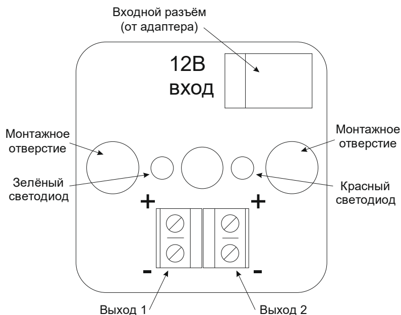
Рисунок 1. Схема подключения устройства GC-0012U3
