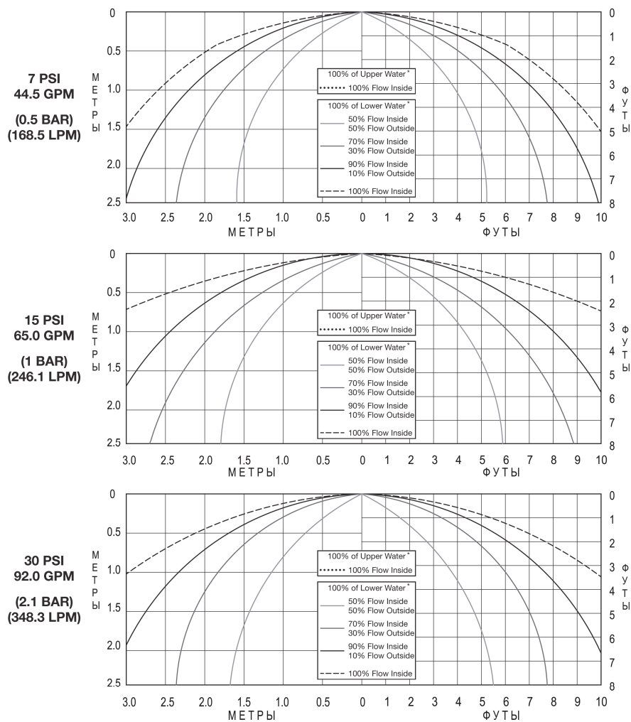
Рис. 6 Карта орошения оросителей модели TY7226 (тип ESFR-17) с плоской розеткой
