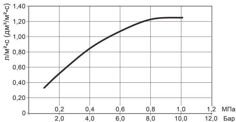
Рис. 9 График зависимости интенсивности орошения оросителей модели TY7126 (тип ESRF-17) от давления (ГОСТ Р 51043-2002)
