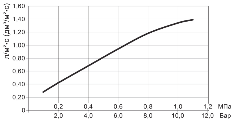
Рис. 7 График зависимости интенсивности орошения оросителей модели TY7226 (тип ESFR-17) от давления (ГОСТ Р 51043-2002)
