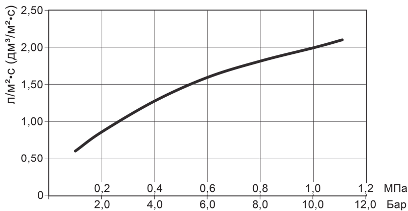
Рис. 11 График зависимости интенсивности орошения оросителей модели TY9226 (тип ESRF-25) от давления (ГОСТ Р 51043-2002)
