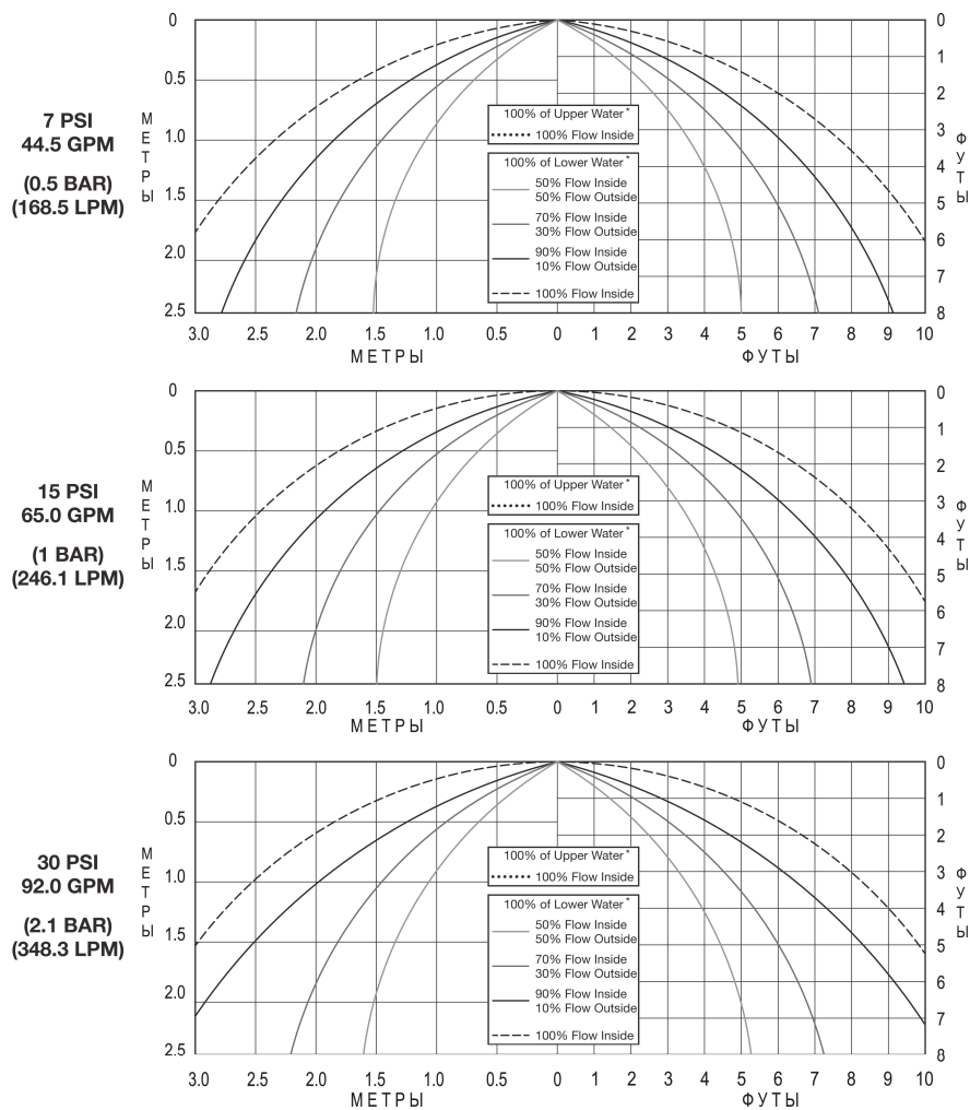
Рис. 8 Карта орошения оросителей модели TY7126 (тип ESRF-17) с вогнутой розеткой
