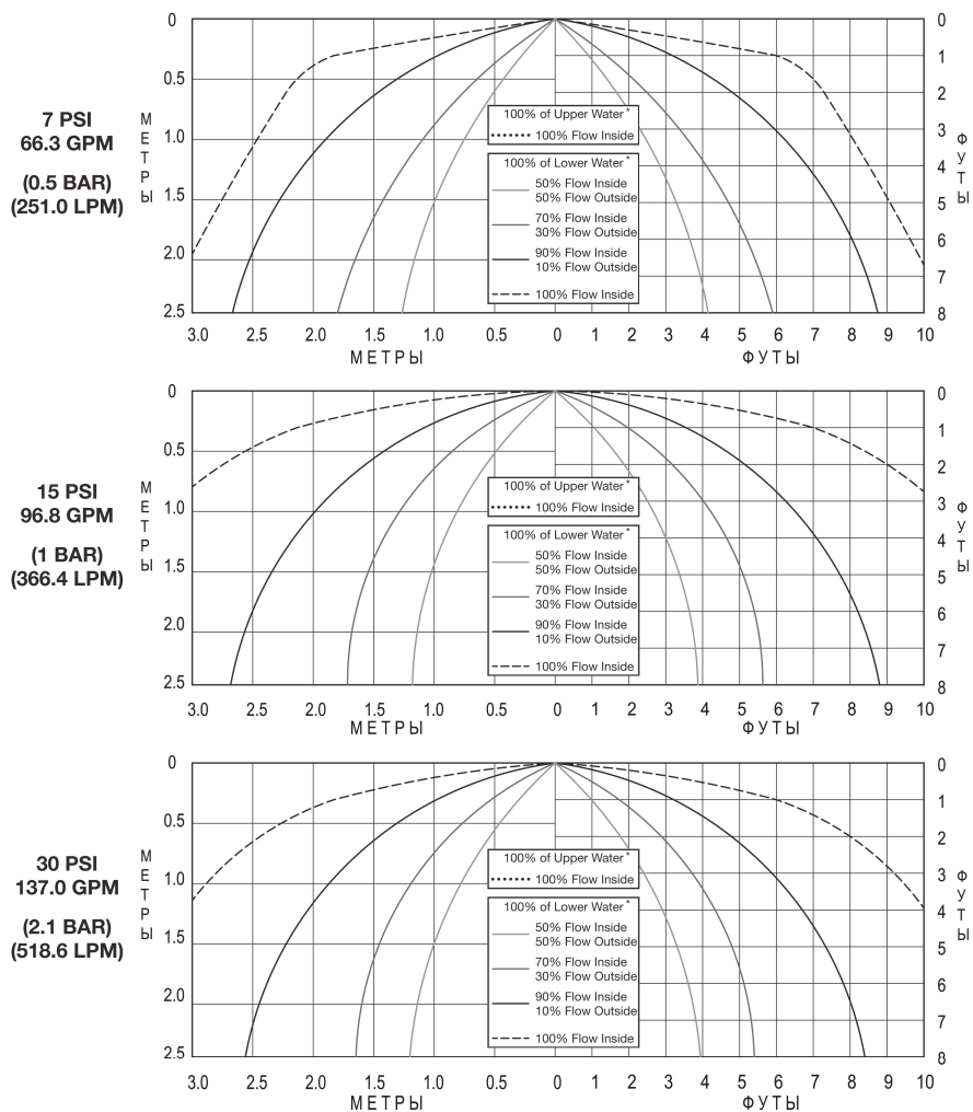
Рис. 10 Карта орошения оросителей модели TY9226 (тип ESRF-25) с плоской розеткой
