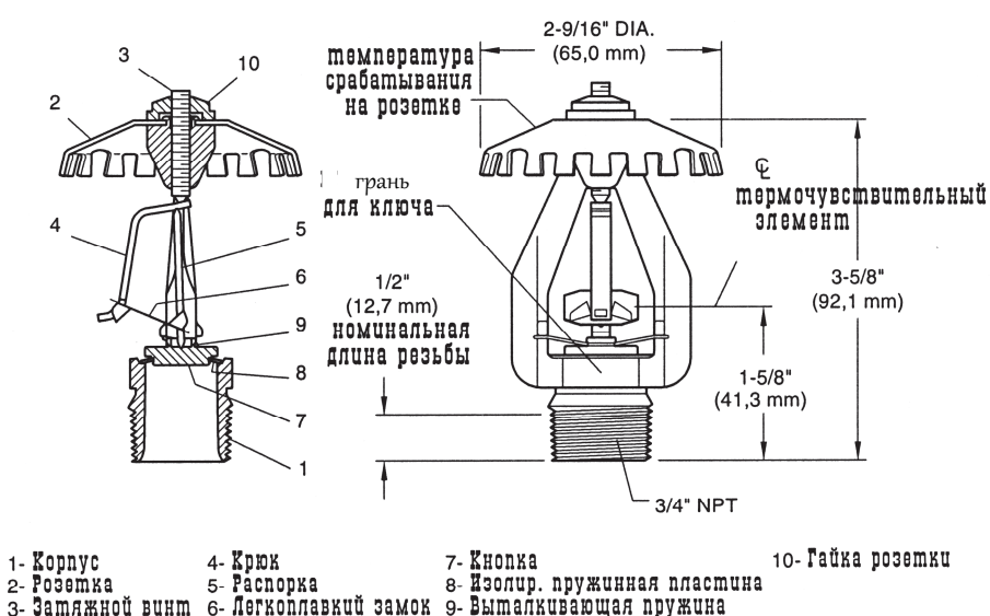
Схема В Быстродействующий спринклерный ороситель для раннего подавления огня ESFR-17 с вогнутой розеткой
