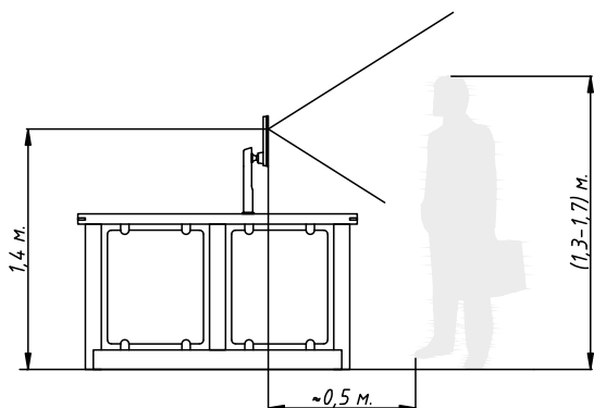
Рис. 6. Рекомендуемое размещение на турникете терминала R20-Face (8T) всех модификаций
