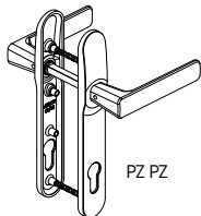
DIN 2750 Handle pair
