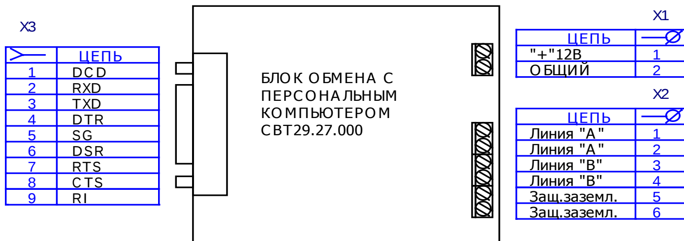
Рис. 3. Клеммные колодки блока обмена с ПК СВТ29.27.000
