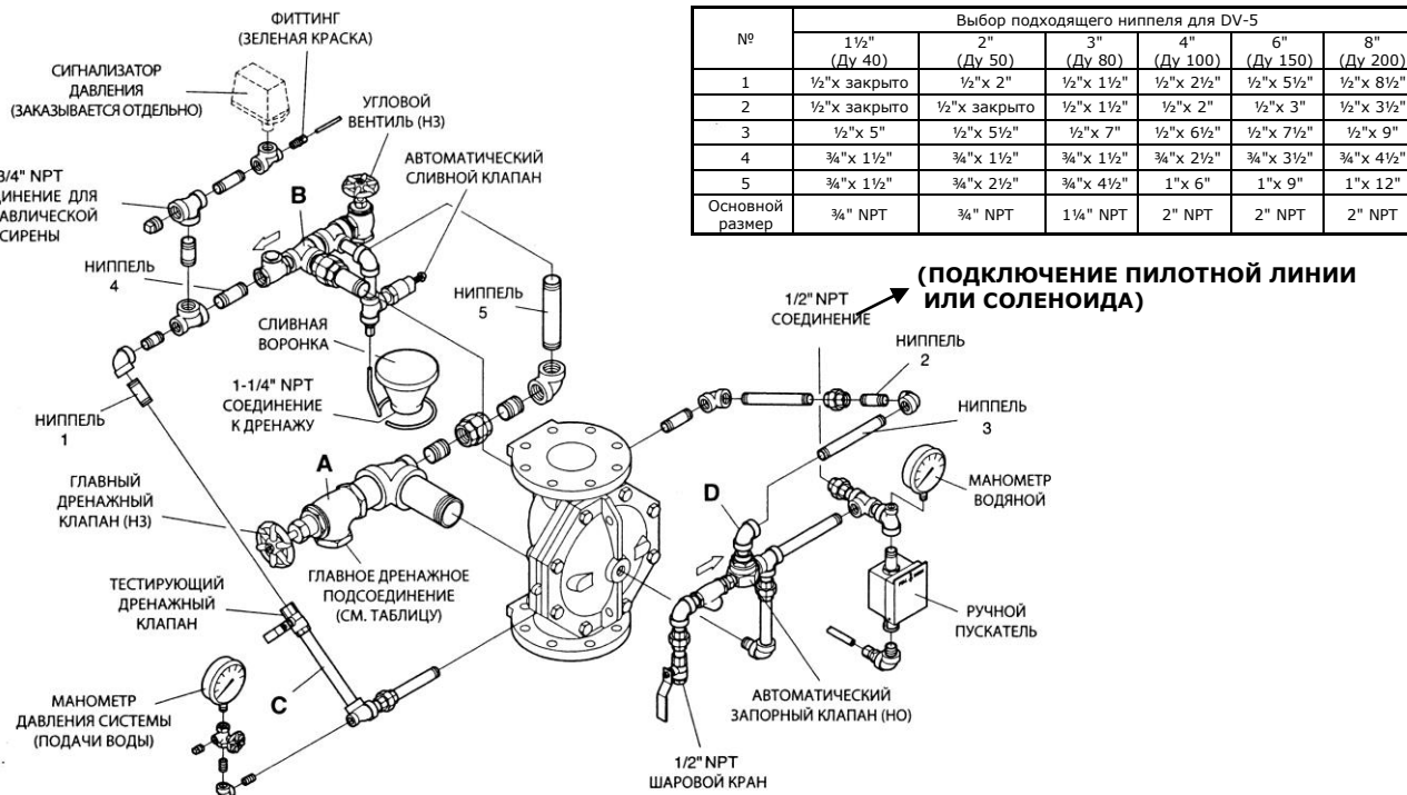
Рис. 5А Клапан объемного тушения модели DV-5 1½"-6" (Ду 40 - Ду 150) - Схема вертикальной сборки «мокрой» обвязки -
