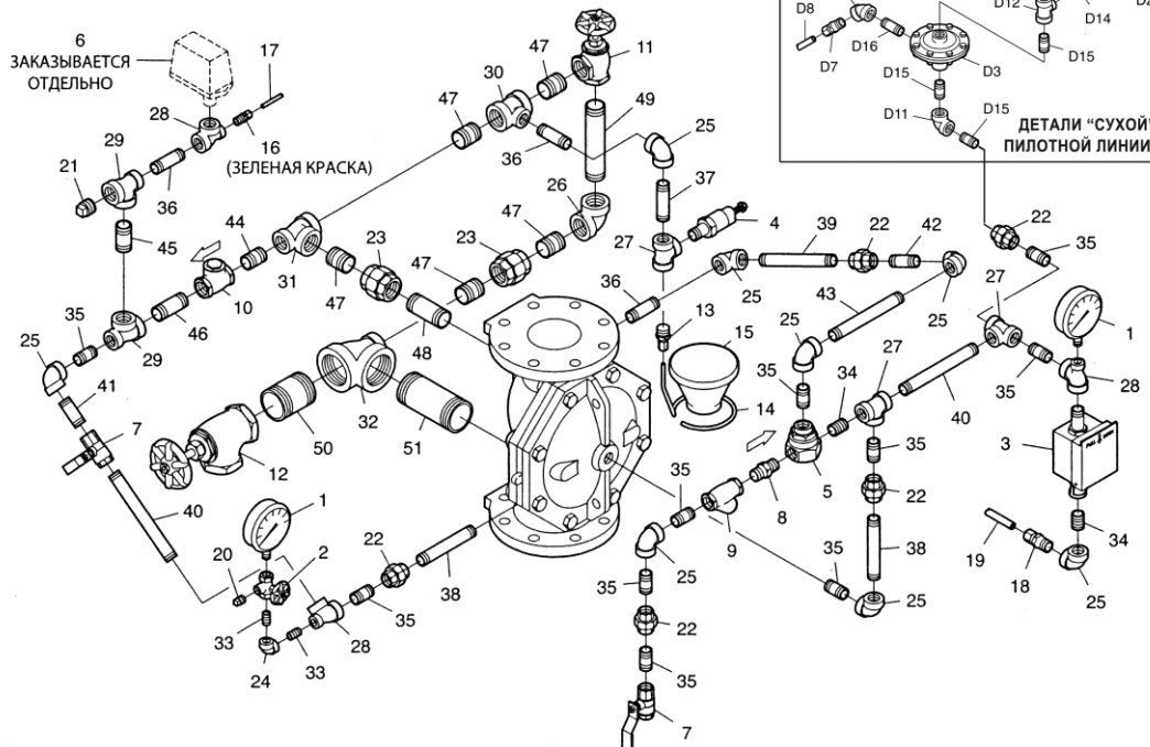
Рис. 4В. Клапан объемного тушения модели DV-5 - Базовая схема обвязки (вертикальная установка) -
