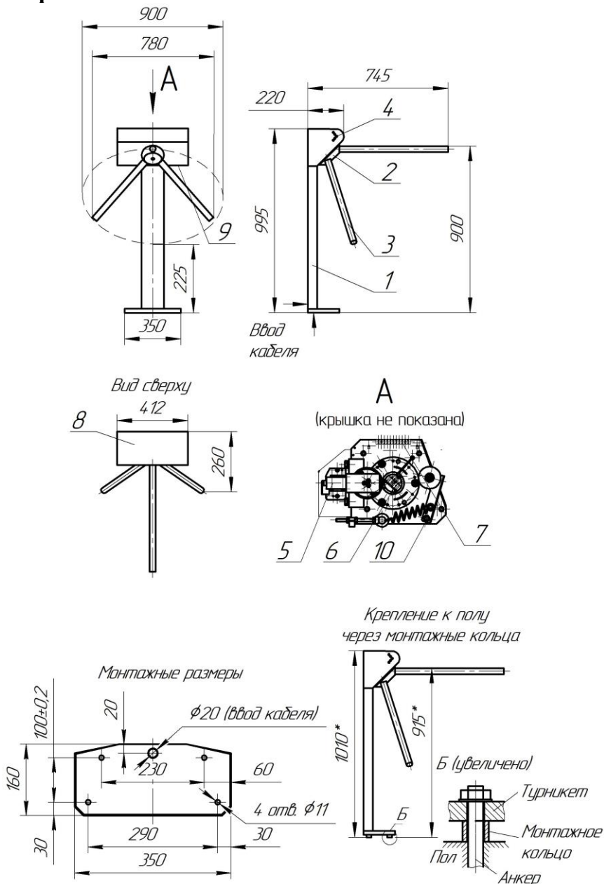
Габаритные и установочные размеры турникетов серии “Ростов-Дон Т9М1-02” (размеры со знаком * - для турникетов с монтажными кольцами)
