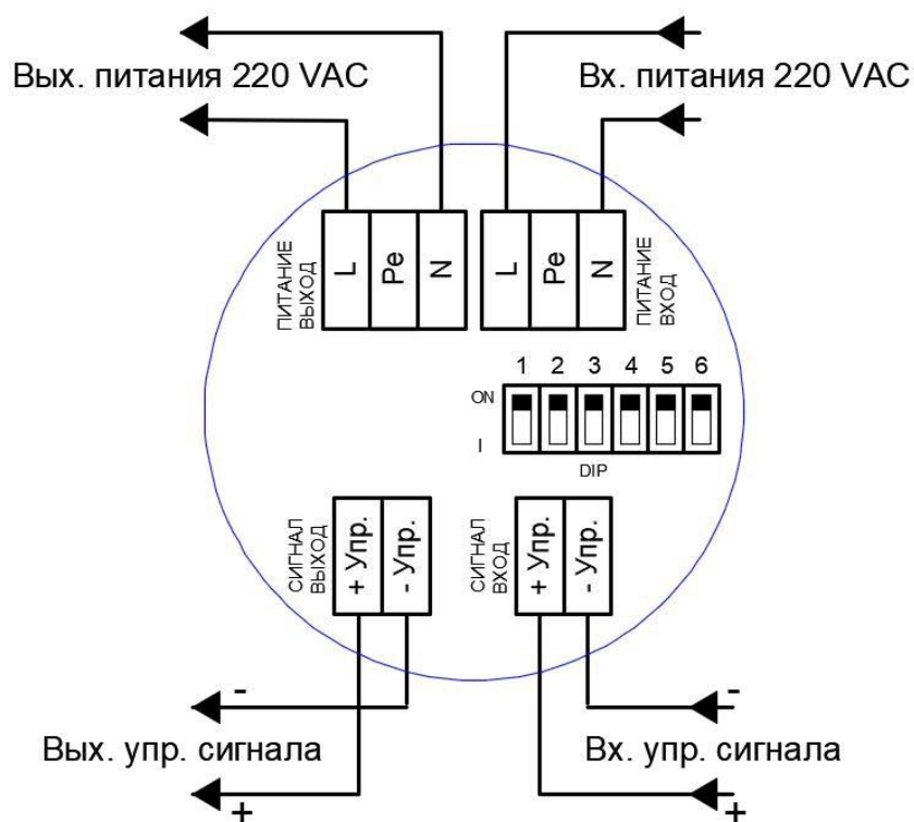
Рис. Б4. Схема четырехпроводного подключения оповещателя 220В АС. Номинал управляющего сигнала: 12÷36В DC, 12÷28В AC.
