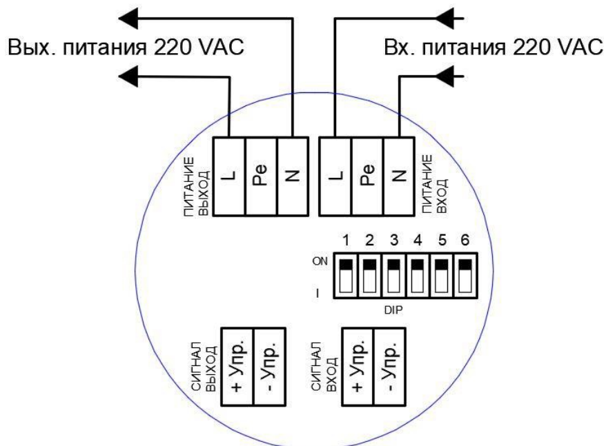
Рис. Б3. Схема двухпроводного подключения оповещателя 220В АС. Номинал управляющего сигнала: 12÷36В DC, 12÷28В AC.
