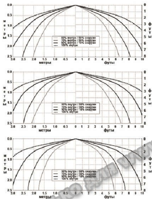
Рис. С Карта орошения оросителей TY4251/TY4231
