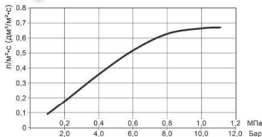
Рис. Е Для оросителей TY4251/TY4231
