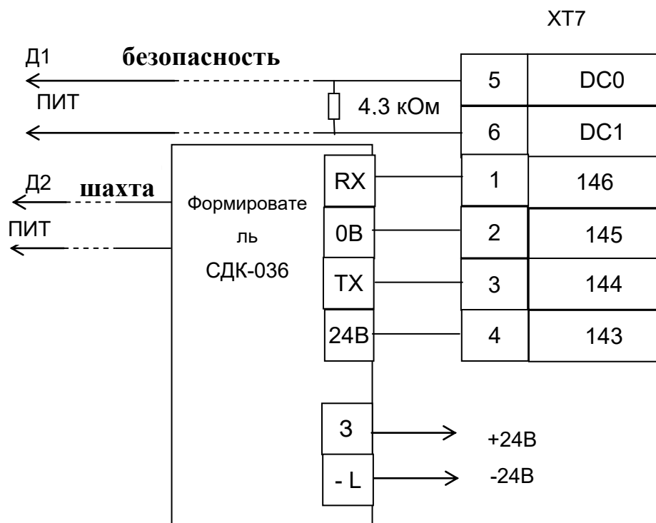
Рис. 11 Подключение к станциям типа УКЛ
