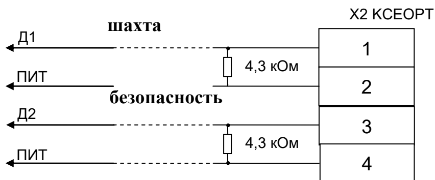
Рис. 13. Подключение для снятия сигнала безопасности и открытия дверей шахты к станции управления фирмы «ОТИС»
