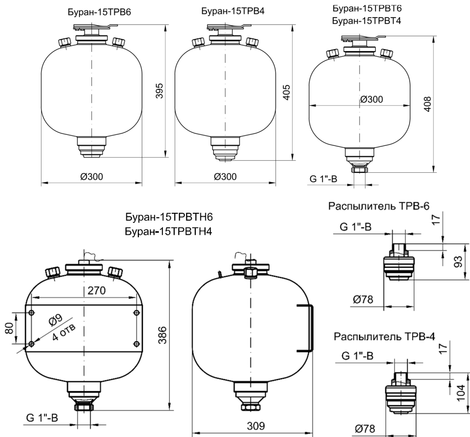
Рис. 1. Габаритные и присоединительные размеры модификаций модулей пожаротушения тонкораспыленной водой «Буран-15ТРВ».
