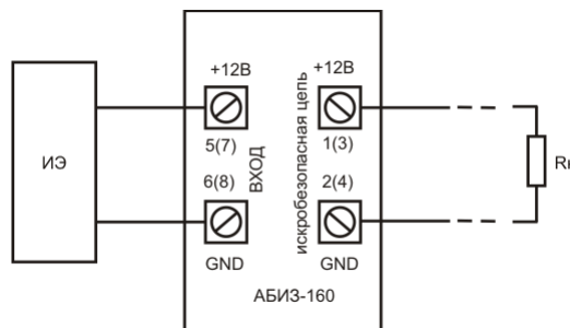
Рис.2 – Клеммные соединения барьера АБИЗ-160.
