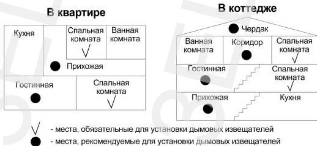
Рисунок 2 – Места установки дымовых извещателей
