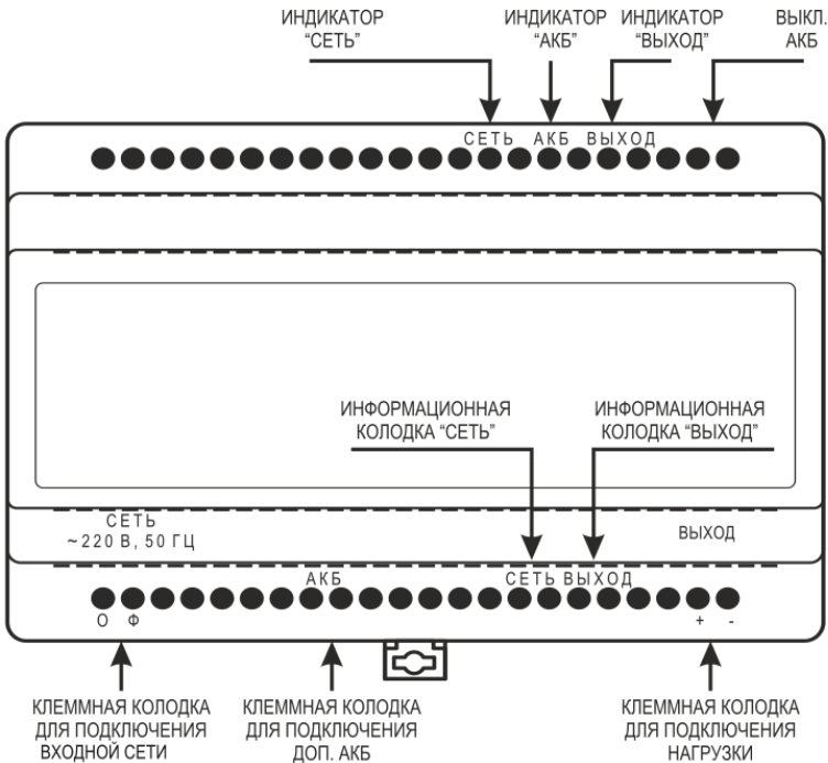
Рисунок 1 – общий вид источника
