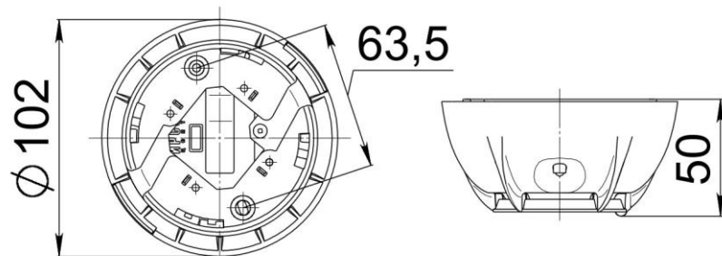
Рисунок 2 – Монтажная схема.
