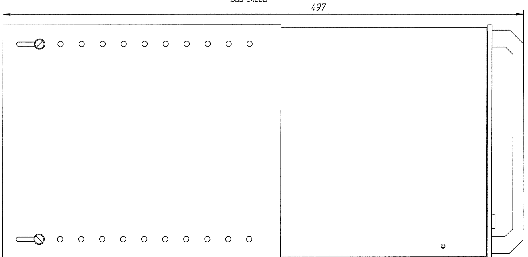
Вид слева
