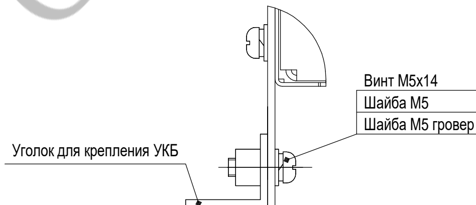
А Крепление уголков к УКБ СГС-22-МЕ300В
