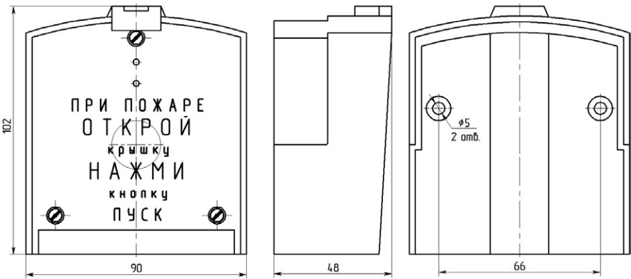
Габаритные и присоединительные размеры пульты ПДП-1 v2 (степень защиты оболочкой IP41)
